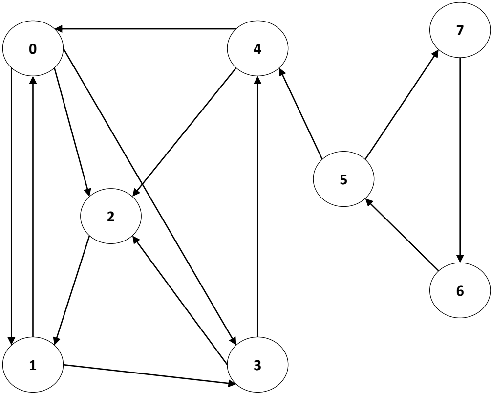
Étape 1: graphe inverse
